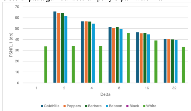
GAMBAR. 6 Pengaruh Delta Terhadap nilai PSNR_1
