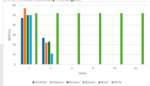
GAMBAR 5. Pengaruh Delta terhadap nilai BER
