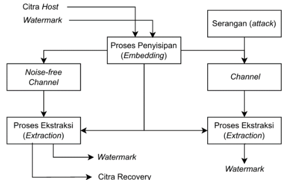
GAMBAR 4. Skema diagram pengujian Sistem Watermarking
