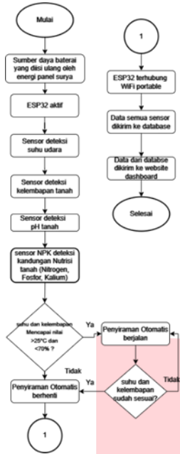
GAMBAR 2. Diagram alur sistem pemantauan
