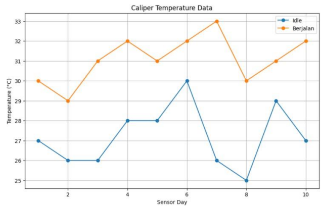
GAMBAR 4.1 Hasil Pengujian Caliper Temperature
