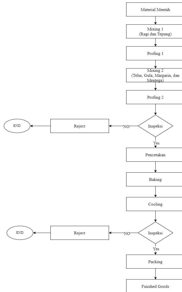
Gambar I. 2 Proses Produksi Roti Bluder
