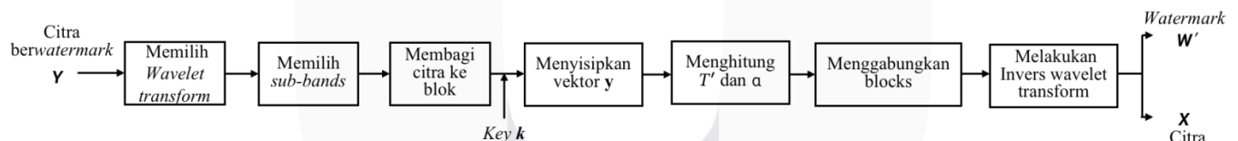
GAMBAR 2 Proses Ekstraksi Watermark
