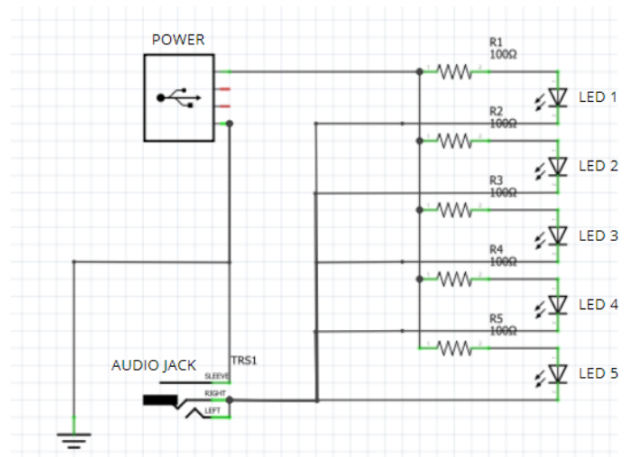
GAMBAR 1. Rangkaian Transmitter
