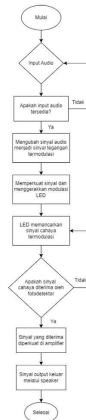
GAMBAR 1. Flowchart Desain Sistem
