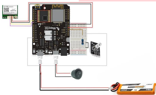
GAMBAR 1. Sistem desain kelistrikan pada Hardware
