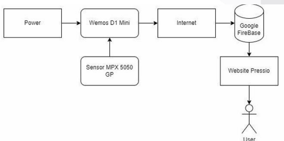
GAMBAR 1 Blok Diagram Desain Sistem
