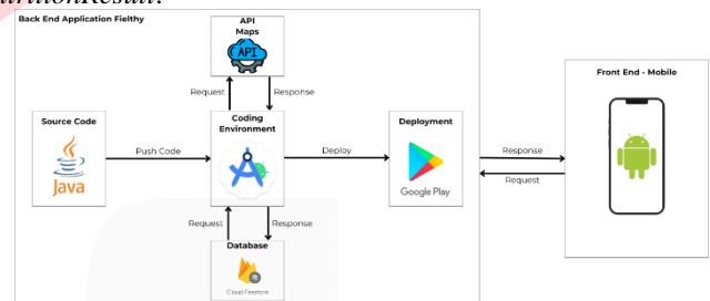
GAMBAR 3 Arsitektur Sistem Aplikasi Fielthy
