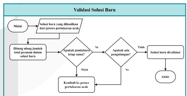
GAMBAR 10 (Diagram Alir Validasi Solusi Baru)
