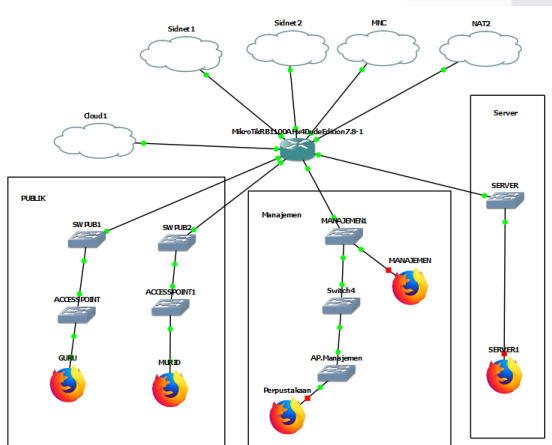
Gambar 9. Topologi Pengujian
