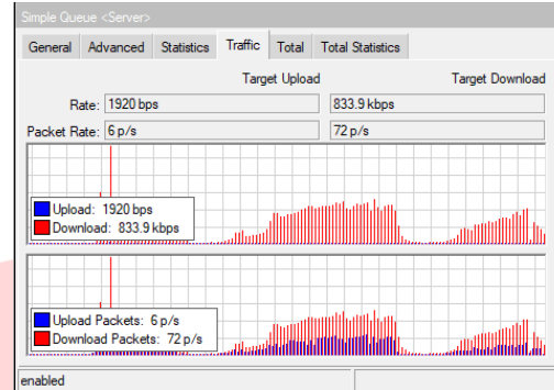
Gambar 14. Hasil tes bandwidth pada switch server di ruang administrasi sebelum dilakukan manajemen bandwidth
