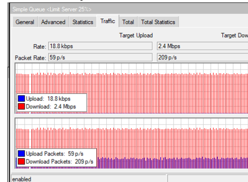
Gambar 15. Hasil tes bandwidth pada switch server di ruang administrasi setelah dilakukan manajemen bandwidth
