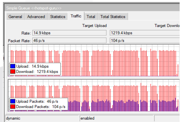
Gambar 23. Hasil tes bandwidth switch publik dengan user guru setelah dilakukan manajemen bandwidth
