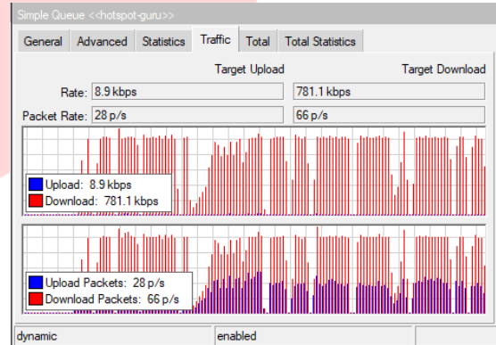
Gambar 22. Hasil tes bandwidth switch publik dengan user guru sebelum dilakukan manajemen bandwidth
