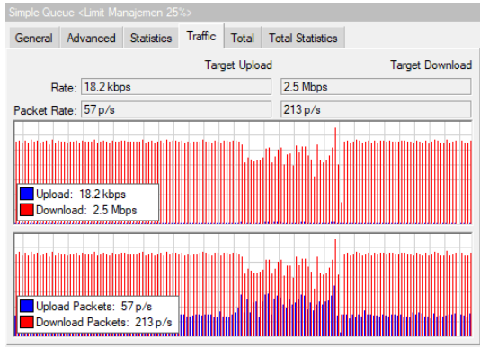
Gambar 17. Hasil tes bandwidth switch manajemen setelah dilakukan manajemen bandwidth
