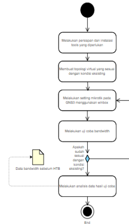
gambar 10. Skenario pengujian kondisi virtual eksisting sebelum dilakukan HTB.
