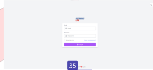
Gambar 10 (Halaman Login)
