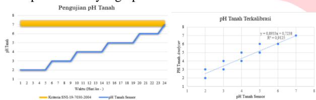
(a) Pengujian pH Tanah, (b) Grafik pH Tanah Terkalibrasi
