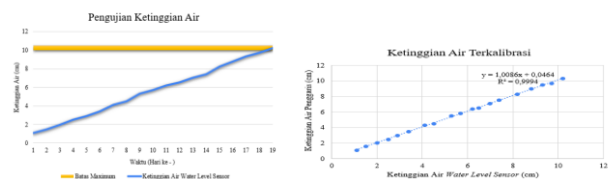
(a) Pengujian Ketinggian Air, (b) Grafik Ketinggian Air Terkalibrasi
