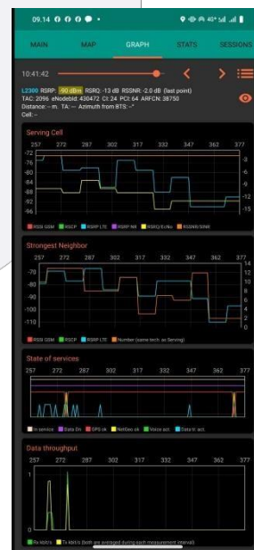
GAMBAR 2: Simulasi Nilai RSRP downlink pada rute Bandung- Rancaekek
