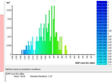
GAMBAR 10b: RSRP Optimasi
