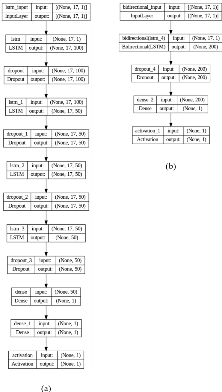
Gambar 4. Arsitektur LSTM (a), Arsitektur BiLSTM (b)
