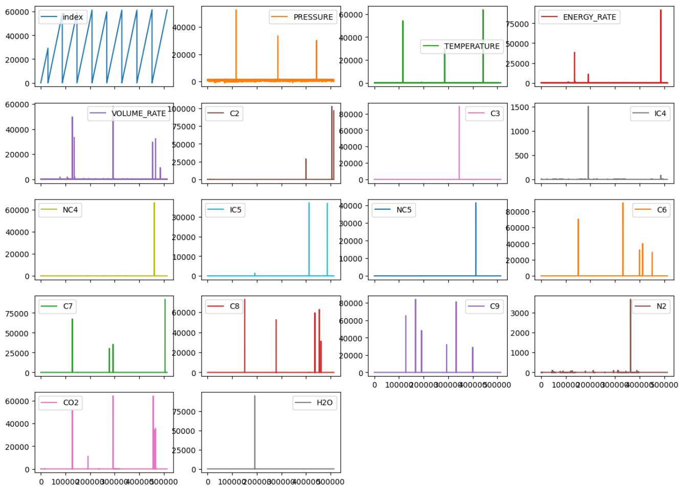
Gambar 6. Visualisasi Trend Dataset
