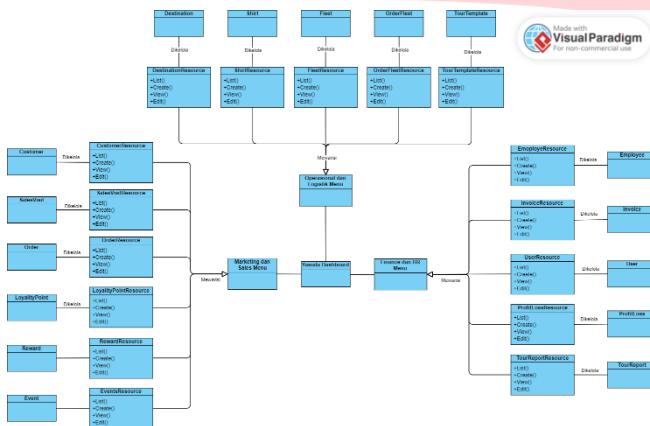
GAMBAR 4 Class diagram Aplikasi Divisi Marketing
