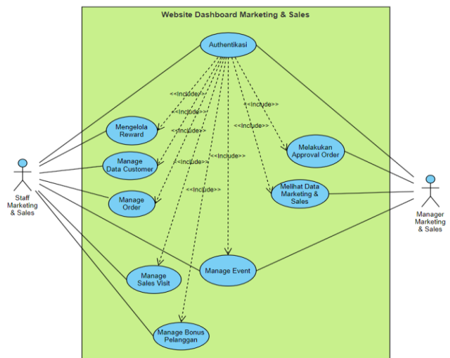
GAMBAR 2 Use Case Diagram Aplikasi Divisi Marketing
