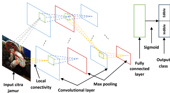
GAMBAR 1 (ARSITEKTUR CNN)
