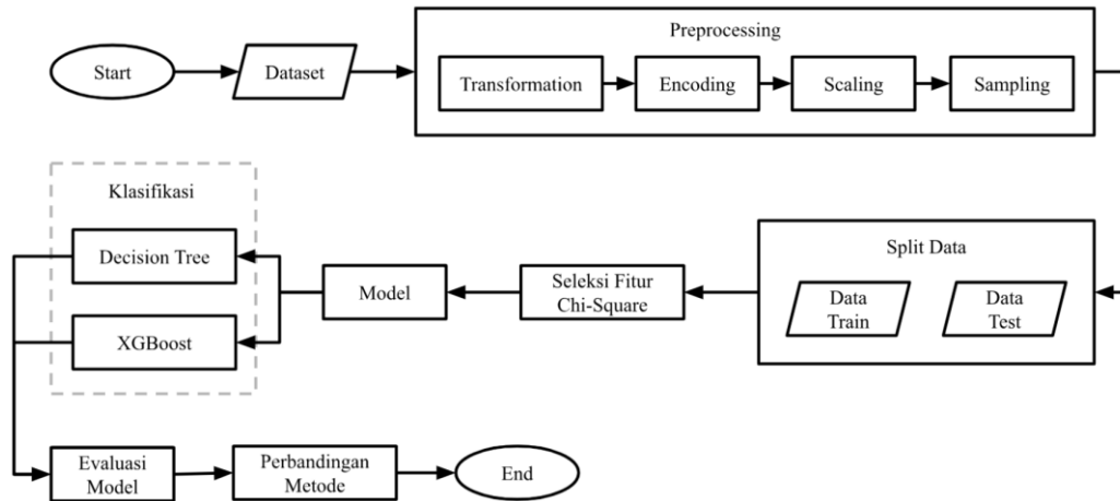
Gambar 1. Flowchart Perancangan Sistem
