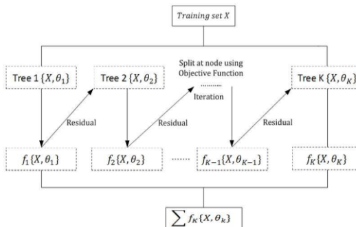
Gambar 3. Arsitektur XGBoost
