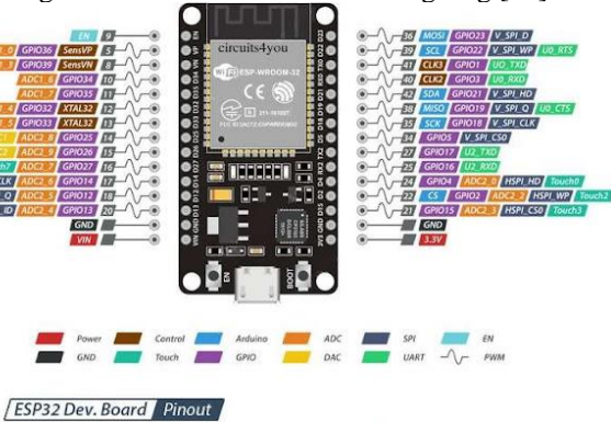
GAMBAR 3 Mikrokontroler ESP-32 [23]
