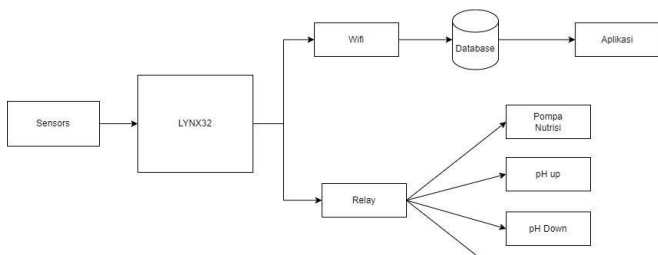
GAMBAR 5 Blok Diagram Otomatisasi
