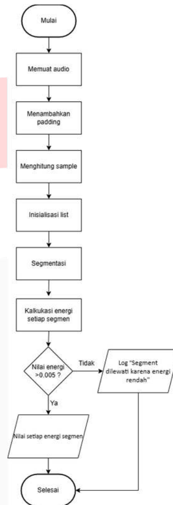
GAMBAR 1 Alur Segmentasi
