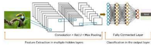
Gambar 5. Ilustrasi Arsitektur CNN
