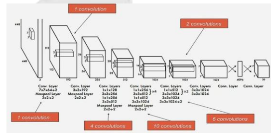
Gambar 6. Ilustrasi Arsitektur YOLO
