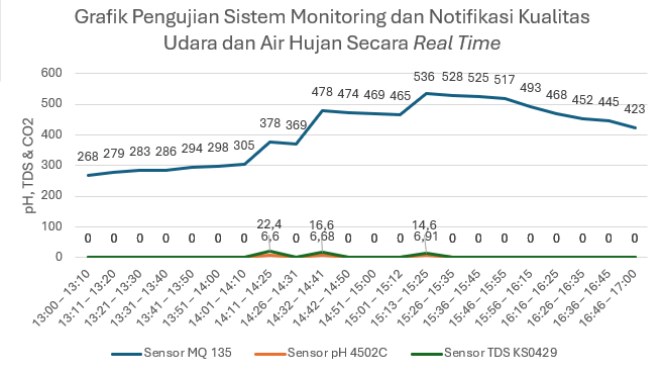
GAMBAR 7(E) PENGUJIAN SISTEM MONITORING DAN NOTIFIKASI KUALITAS UDARA DAN AIR HUJAN SECARA REAL-TIME
