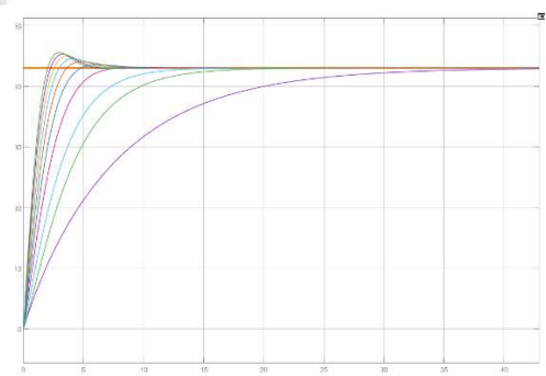
GAMBAR 10 (HASIL PENALAAN SISTEM DENGAN PENGENDALI PID PADA SIMULINK DI TIPE LAPTOP KASUAL (METODE TRIAL ERROR ))
