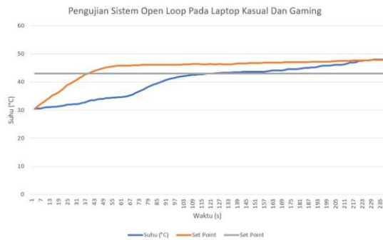
GAMBAR 8 (HASIL PENGUJIAN SISTEM OPEN LOOP PADA LAPTOP KASUAL DAN GAMING )
