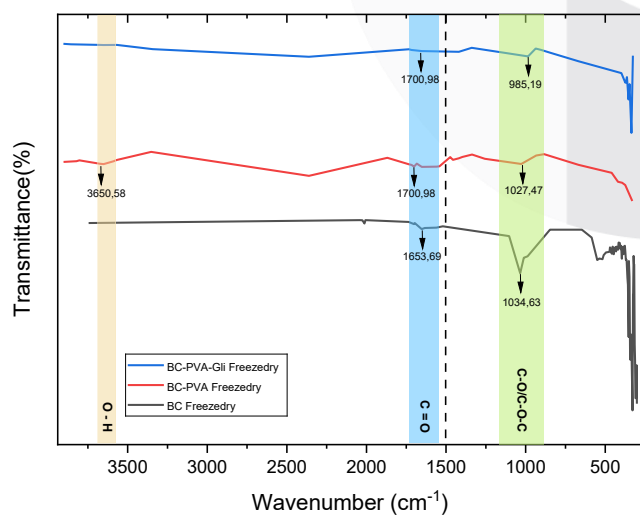
GAMBAR 5 (PERBANDINGAN SPEKTRA IR SAMPEL FREEZE-DRYING)
