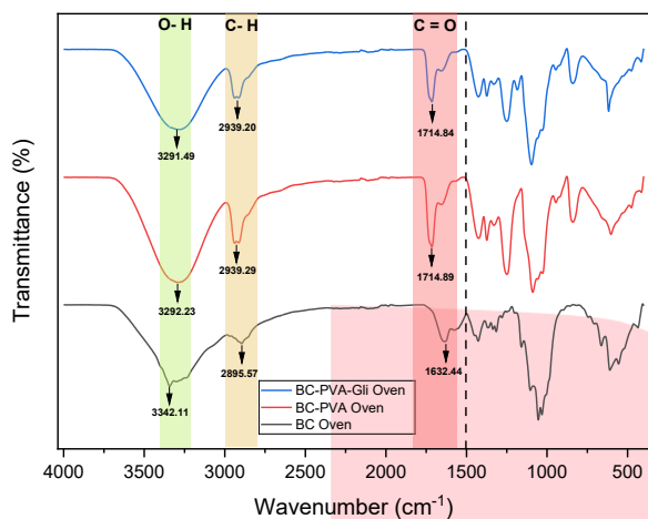
GAMBAR 4 (PERBANDINGAN SPEKTRA IR SAMPEL OVEN-DRYING)
