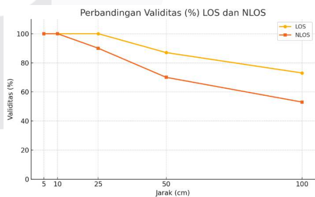
GAMBAR 8 HASIL PENGUJIAN VALIDITAS PERANGKAT LI-FI
