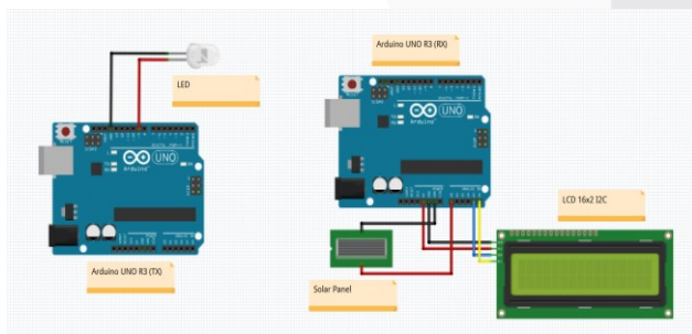
GAMBAR 4 ARSITEKTUR SISTEM
