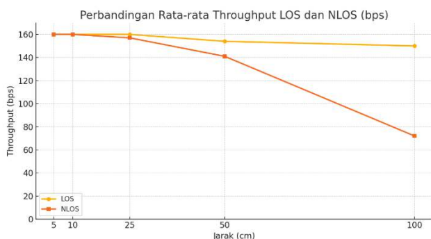
GAMBAR 9 HASIL PENGUJIAN THROUGHPUT
