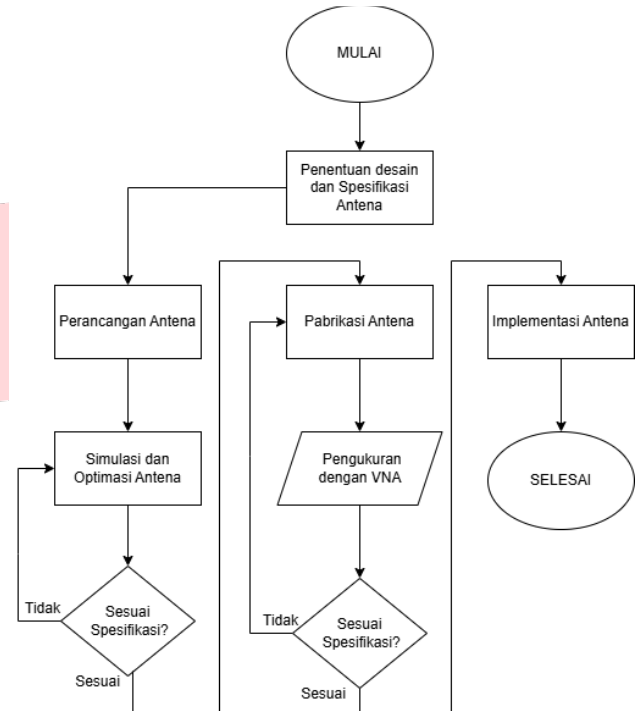
GAMBAR 1 Diagram perancangan Antena Mikrostrip Array
