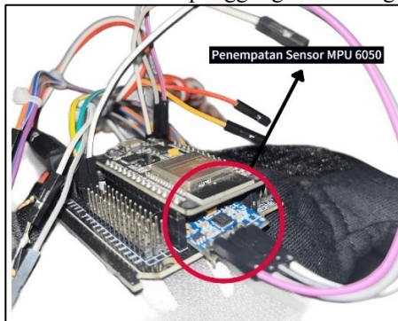
GAMBAR 5 (PELETAKAN MPU PADA SARUNG TANGAN)
