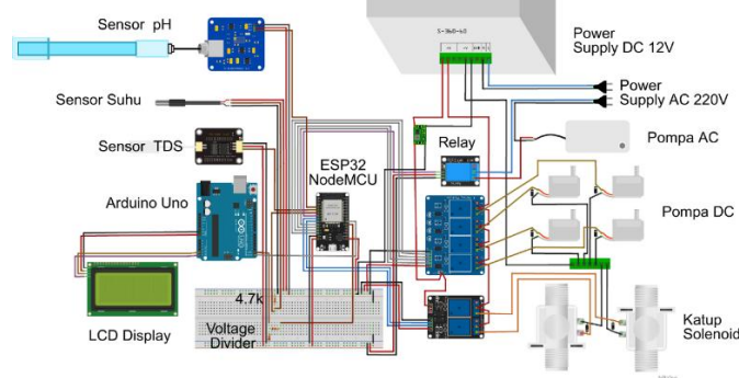
Gambar 2. Wiring Perangkat IoT
