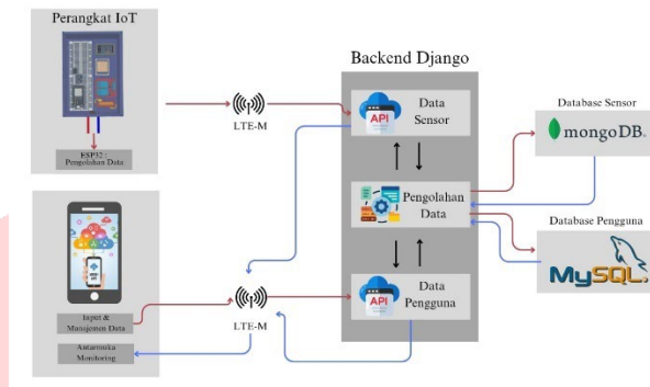
GAMBAR 1 Desain sistem
