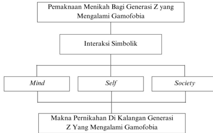
Gambar 2 1Kerangka Pemikiran
