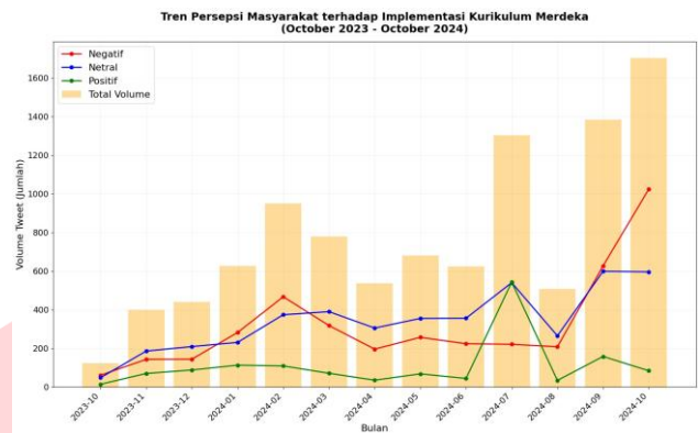
Visualisasi Perkembangan Tren dari setiap Sentimen
