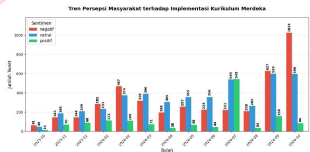
Visualisasi Perkembangan Tren dari setiap Sentimen
