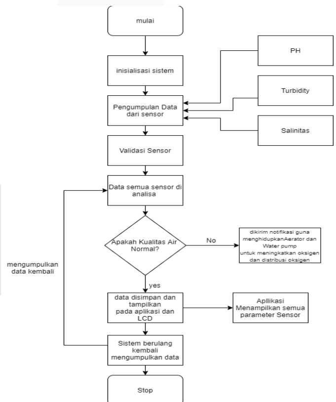
GAMBAR 5 (ALUR KERJA SISTEM)
