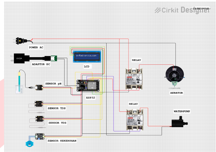
GAMBAR 4 (DESAIN ALAT)
