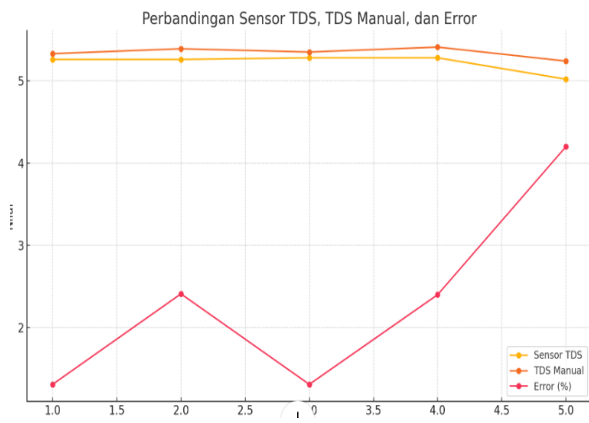
GAMBAR 10 (GRAFIK PERBANDINGAN SENSOR TDS, TDS MANUAL DAN ERROR)
