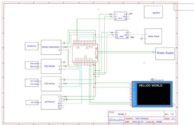
GAMBAR 3 (DESAIN SISTEM)
