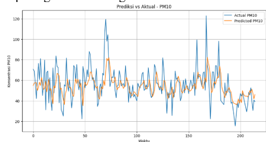
GAMBAR 5. Prediksi dan Aktual PM10 Model LSTM
