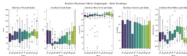
GAMBAR 2. Visualisasi BoxPlot
