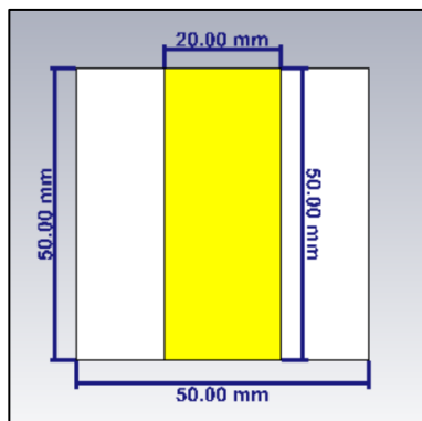
Gambar 3 (Tampak belakang tampilan layer 1 antenna DGS dengan Double Layer)
