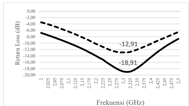
Gambar 13 (perbandingan return loss simulasi dan pengukuran)
