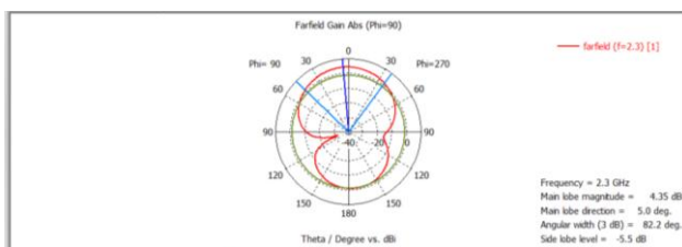
Gambar 11 (Hasil pola radiasi rancangan antenna)
