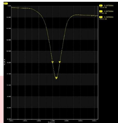
Gambar 12 (Hasil return loss pengukuran antenna)
