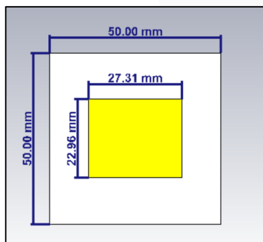
Gambar 4 (Tampak depan tampilan layer 2 antenna DGS dengan Double Layer)
