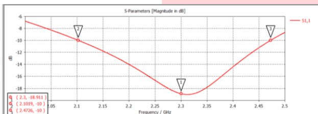
Gambar 9 (Hasil return loss dan bandwidth rancangan antenna)
