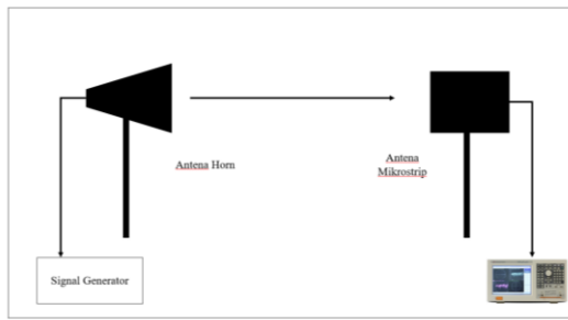
Gambar 8 (Ilustrasi Pengukuran gain dan pola radiasi Antena)
