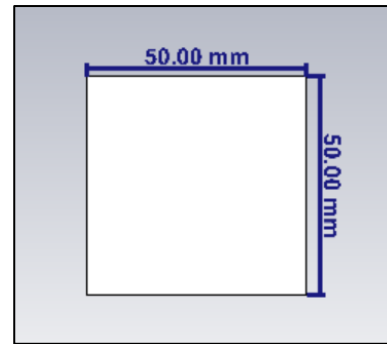
Gambar 5 (Tampak belakang tampilan layer 2 antenna DGS dengan Double Layer)
