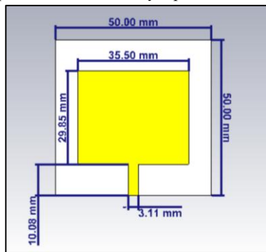
Gambar 2 (Tampak depan tampilan layer 1 antenna DGS dengan Double Layer)
