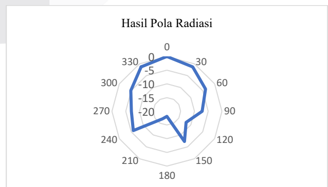
Gambar 14 (Hasil pola radiasi pengukuran antenna)
