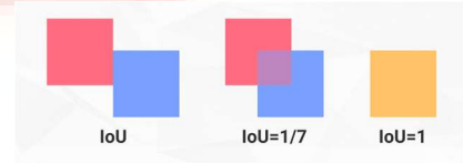
Gambar 2 Ilustrasi Nilai IoU[13]
