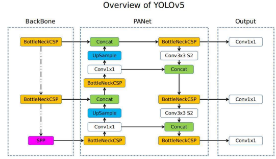
Gambar 1 Cara Kerja YOLOv5 [11]
