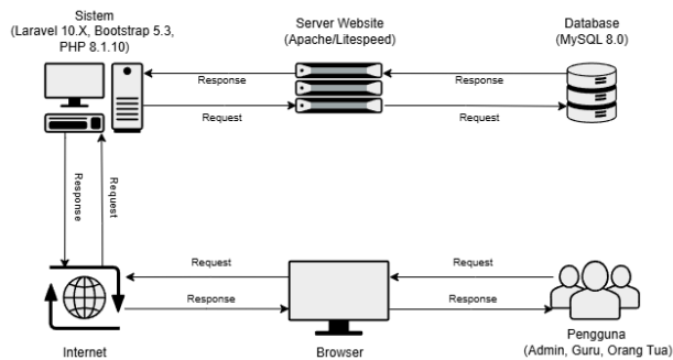
Gambar D (Arsitektur Sistem)
