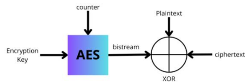
Gambar 3 Algoritma Enkripsi AES
