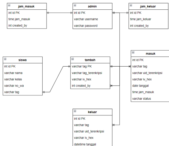
Gambar 7 ERD
