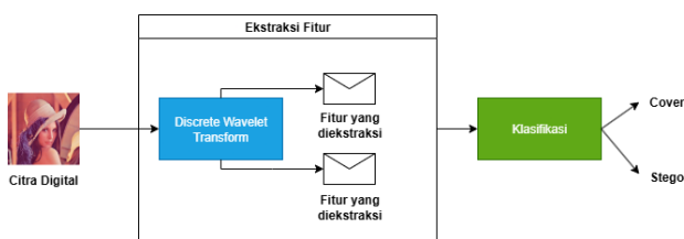
Gambar 1 Alur Proses Steganalisis
