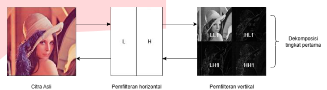
Gambar 2 Cara Kerja DWT
