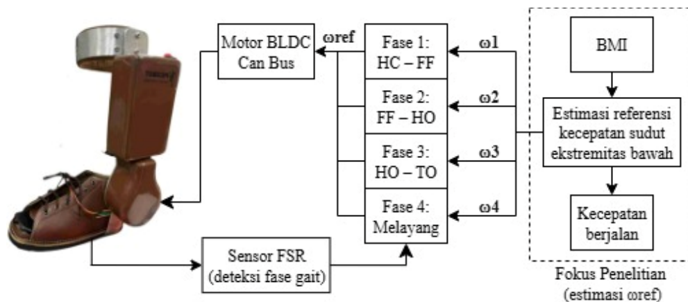
Gambar I. 1 Integrasi Parameter Kontrol Kecepatan Sudut Ekstremitas Bawah pada Sistem Picobot
