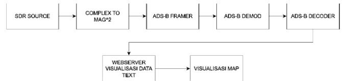
GAMBAR 3 Alur Pemrosesan Sinyal ADS-B
