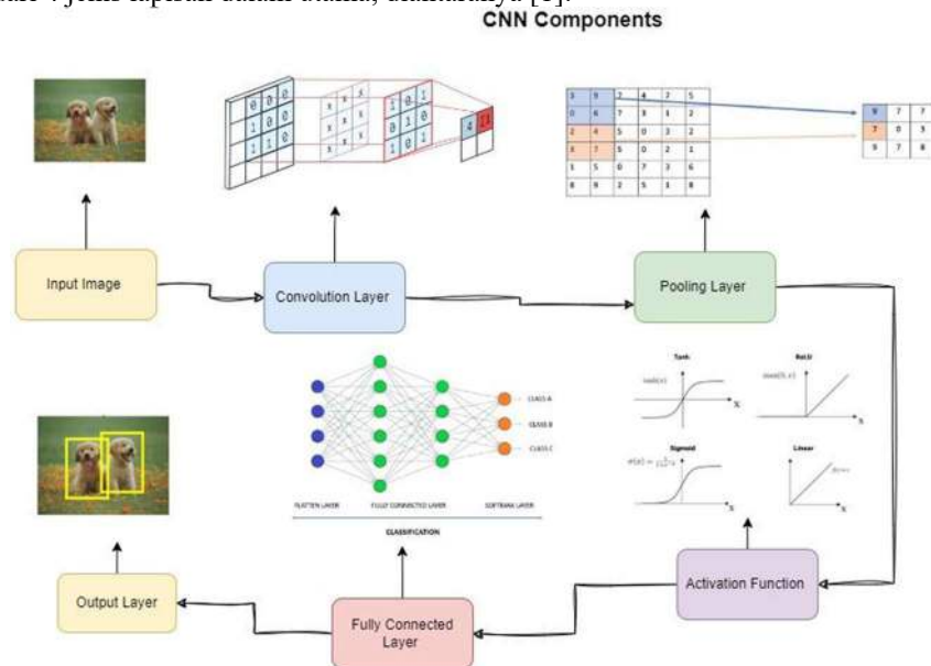
Gambar 1: Ilustrasi Komponen Arsitektur Dasar CNN
