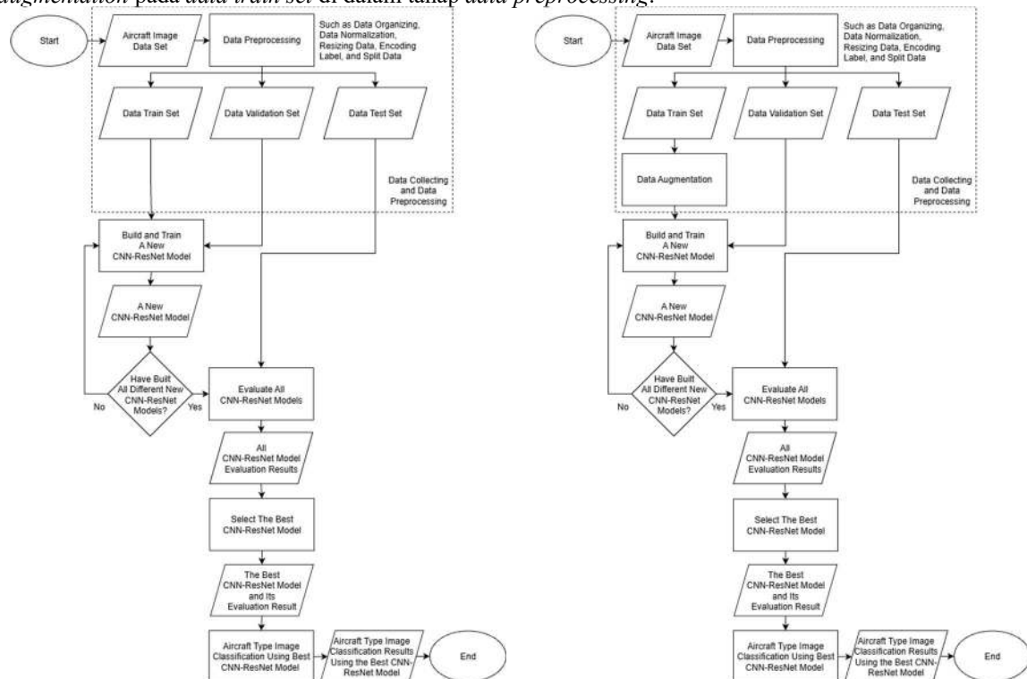
Gambar 3: Flowchart Klasifikasi Citra Pesawat-Skenario 1 Gambar 4: Flowchart Klasifikasi Citra Pesawat-Skenario 2
