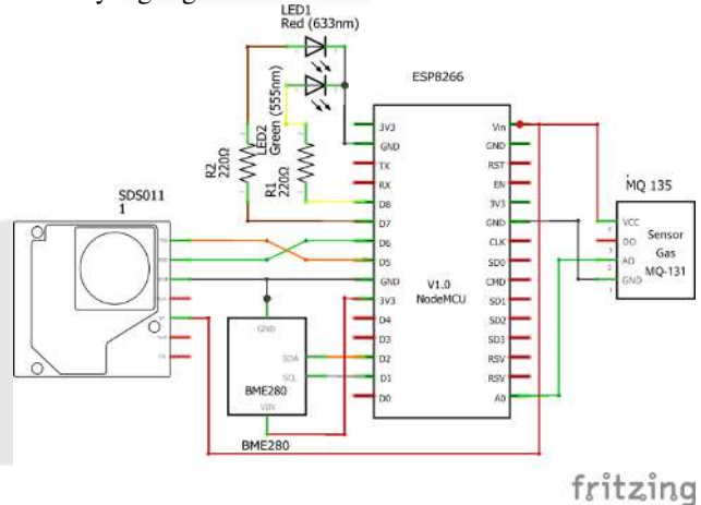
Gambar 2. Skema Sensor
