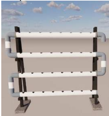
GAMBAR 5 Hidroponik DFT
