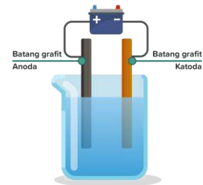
GAMBAR 3 Sistem Elektrolisis
