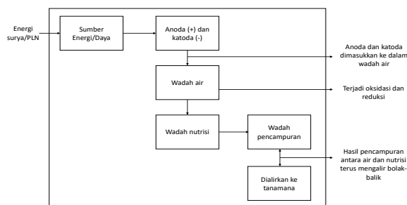
GAMBAR 6 Blok Diagram Elektrolisis
