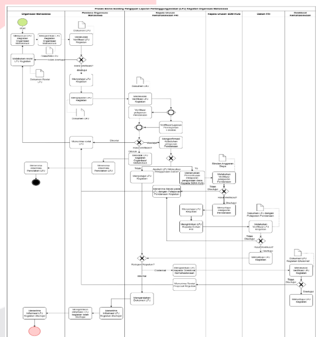
GAMBAR 5 (Proses Bisnis Existing Pengajuan LPJ Kegiatan organisasi Mahasiswa)
