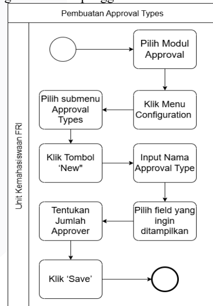
GAMBAR 9 (Alur Pembuatan Master Data Approval Types )
