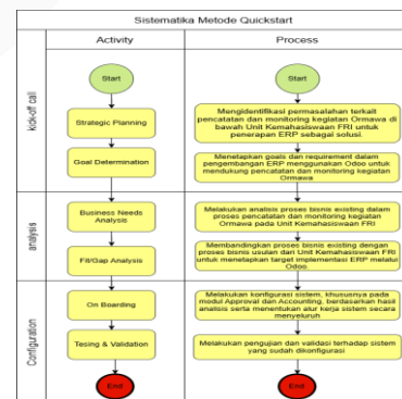
GAMBAR 3 (Sistematika Penyelesaian Masalah)
