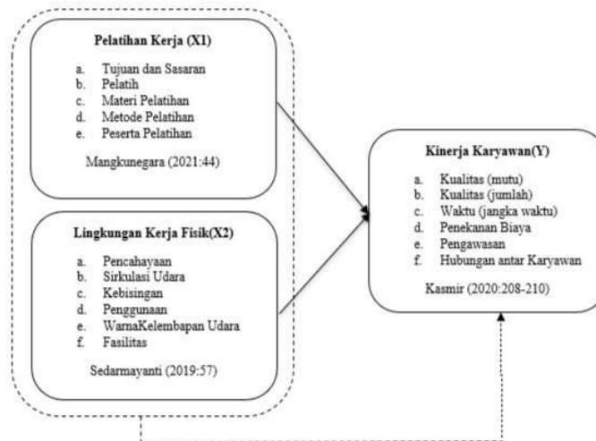
Gambar 1. Kerangka Pemikiran
