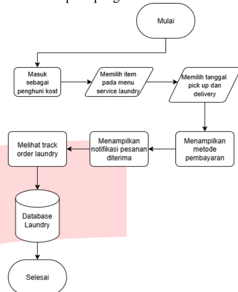
GAMBAR 2 Flowchart Layanan Laundry (Penghuni Kost)
