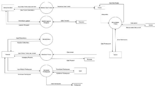
Gambar 2 DFD
