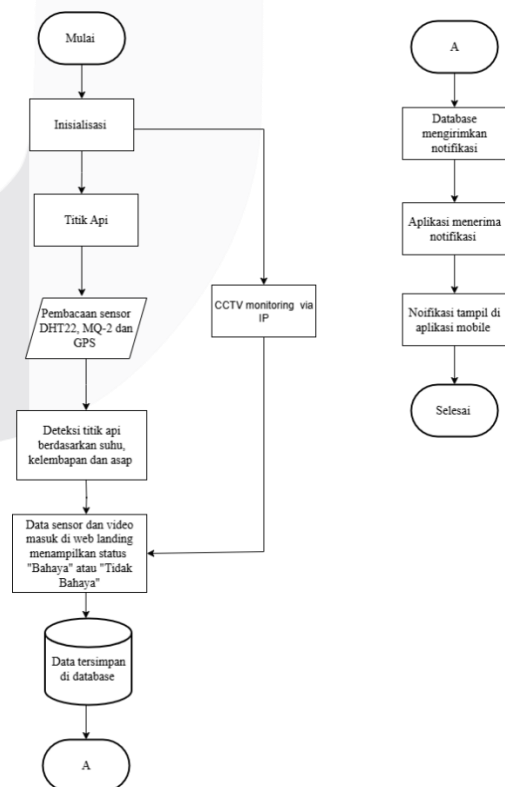
Gambar 7. Flowchart Alur Kerja Sistem
