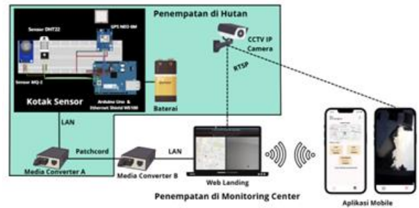
Gambar 6. Blok Diagram Sistem
