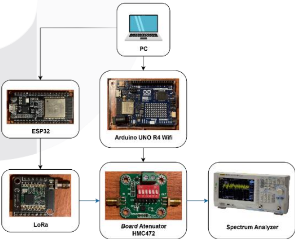
GAMBAR 11 SKENARIO PENGUJIAN BOARD ATENUATOR
